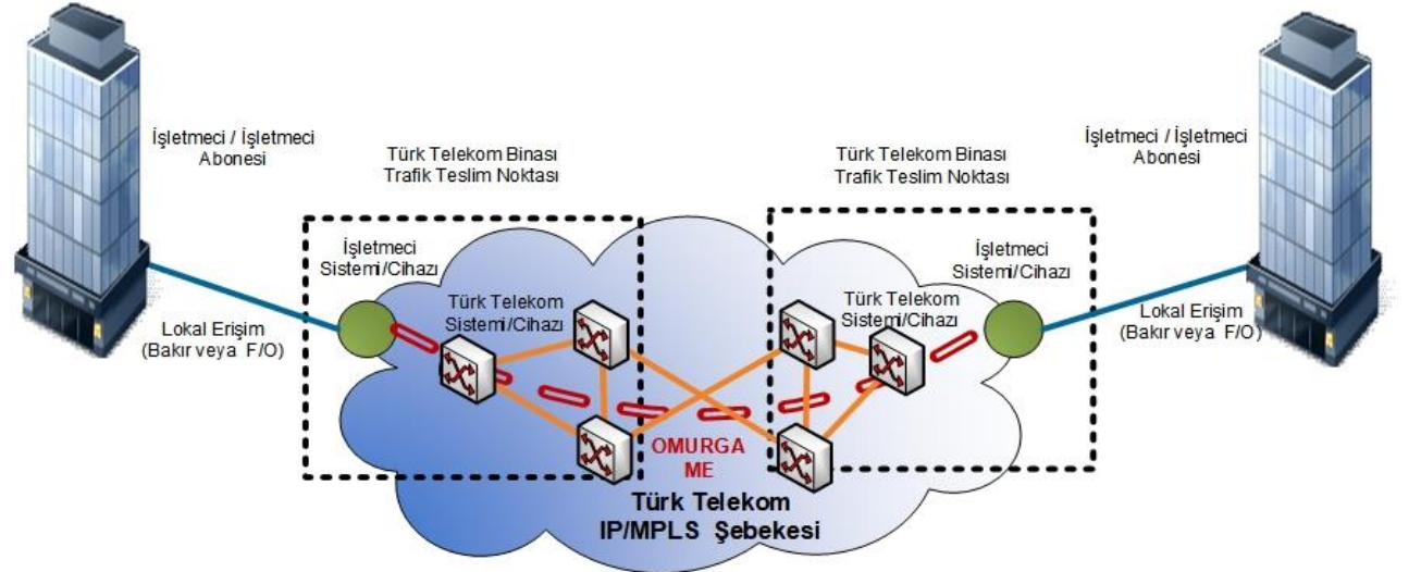
Şekil-11: Omurga ME Şebekesi
