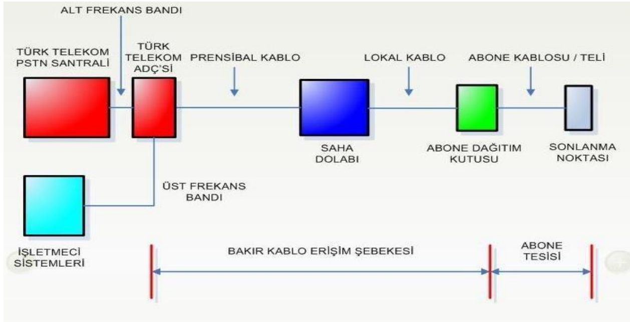
ŞEKİL-3a: Yerel Ağa Ayırıştırılmış Paylaşımlı Erişim Hizmeti
