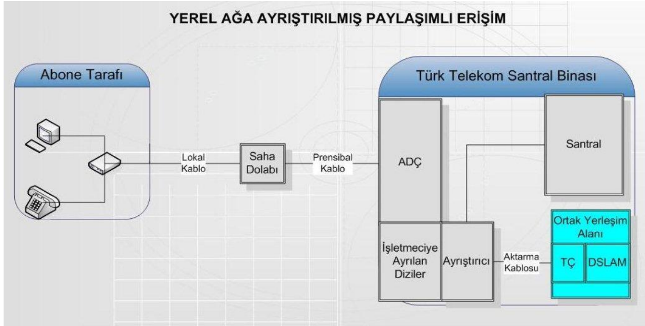
ŞEKİL-3b: Yerel Ağa Ayırıştırılmış Paylaşımlı Erişim Hizmetine ilişkin Ortak Yerleşim Planı
