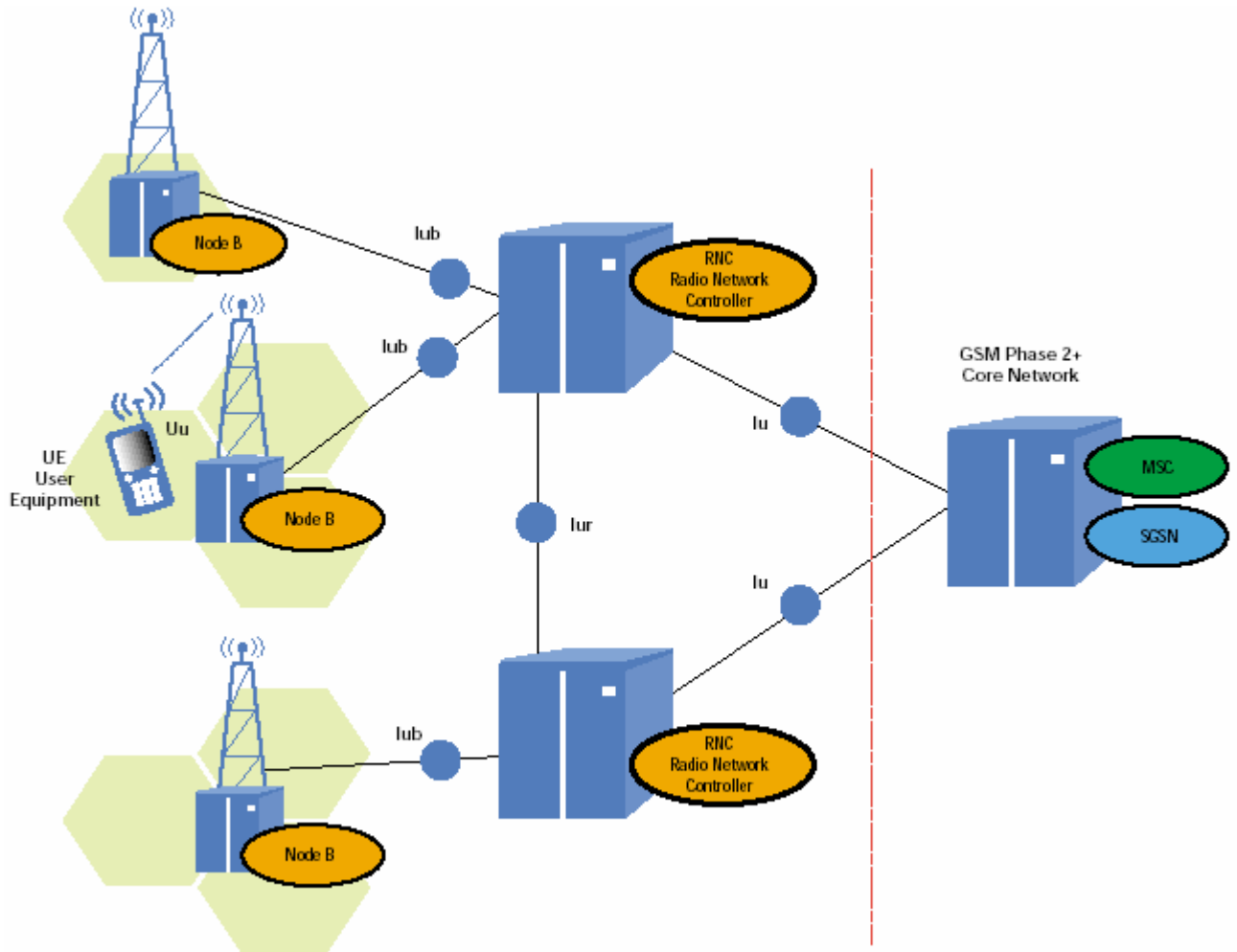
Şekil 22. UTRAN Mimarisi
