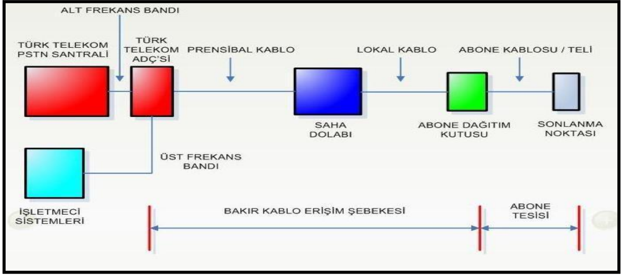
Şekil 6: Yerel Ağa Paylaşımlı Erişim
