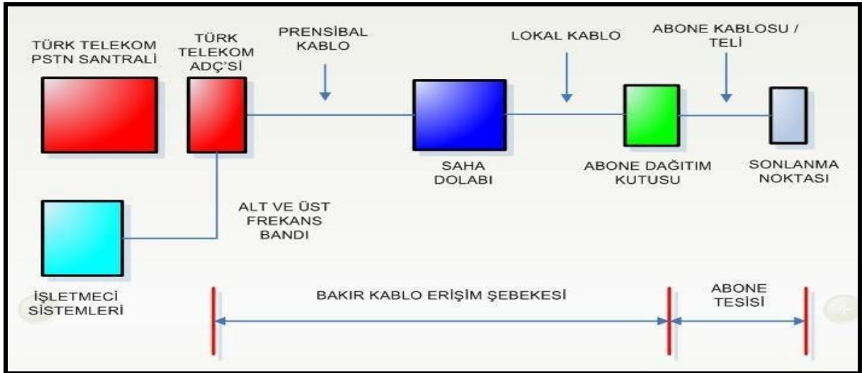
Şekil 5: Yerel Ağa Ayırıştırılmış Tam Erişim
