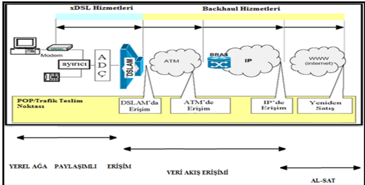
Şekil 12: xDSL Teknolojisine Göre Veri Akış Erişimi
